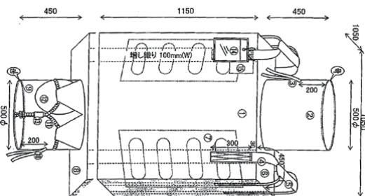
↑ 1200kgコンテナの展開図
